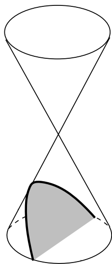
Parabola
