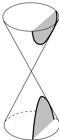
Hyperbola
